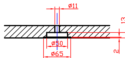
SECCION A - B
